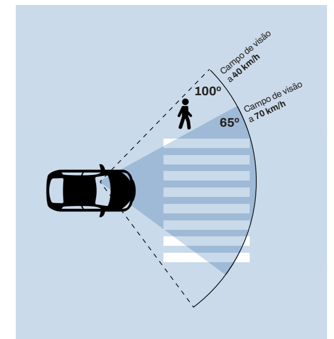
Figura 2 – Redução do campo de visão do condutor conforme o aumento da velocidade.
