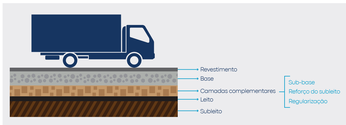
FIGURA 11 Disposição das camadas de pavimento tipo flexível
